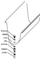
滴水頭上防水板接合示意圖
