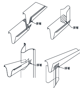
止水板之接合圖
