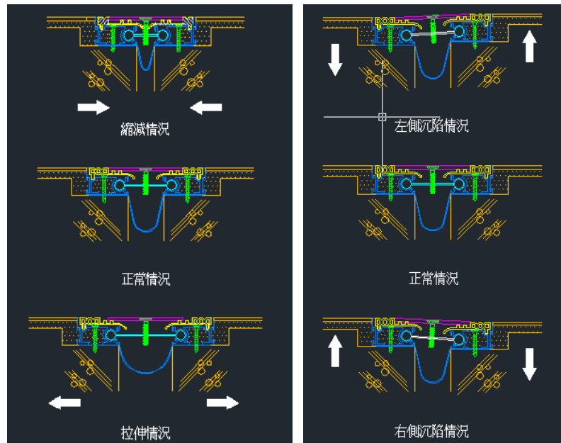
Type 1A 地坪-平面型
