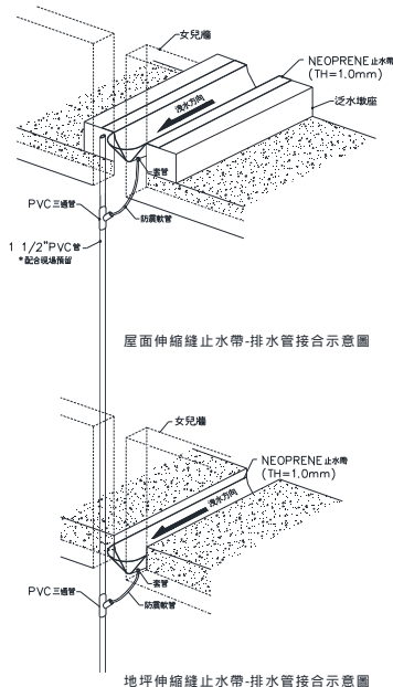
地面伸縮縫止水帶-排水管接合示意圖
